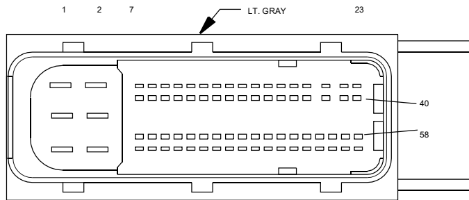
MODULE-POWERTRAIN CONTROL C1 (6.7L)
